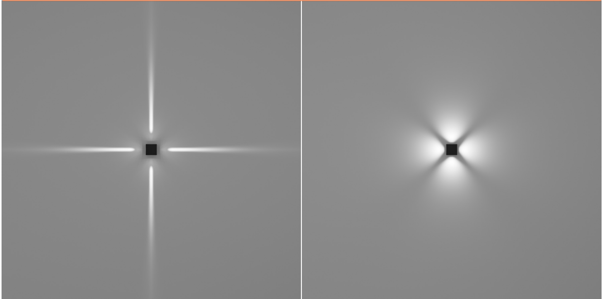
Narrow Beam 3°
