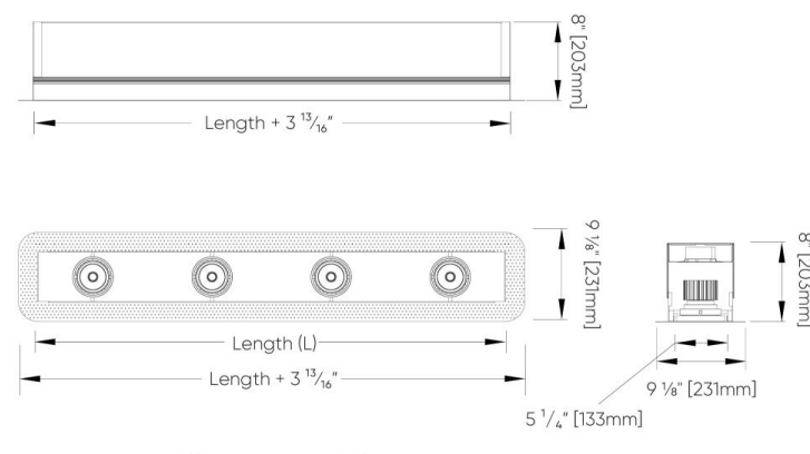
Trimless - no trim (TN)
