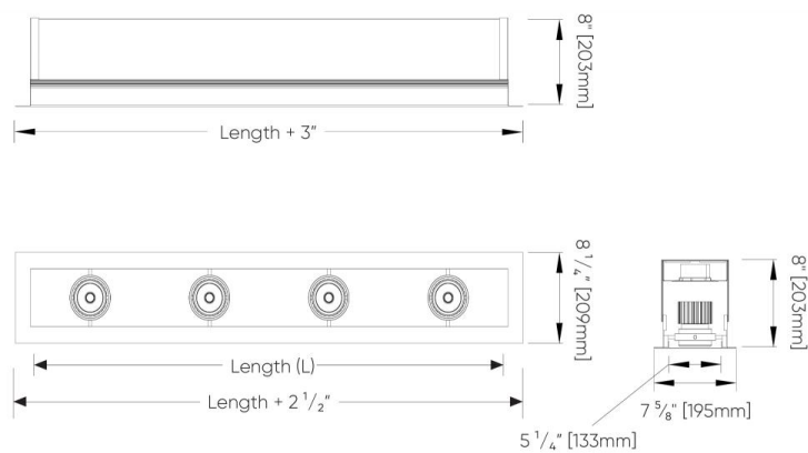
Bezel Trim (TY)
