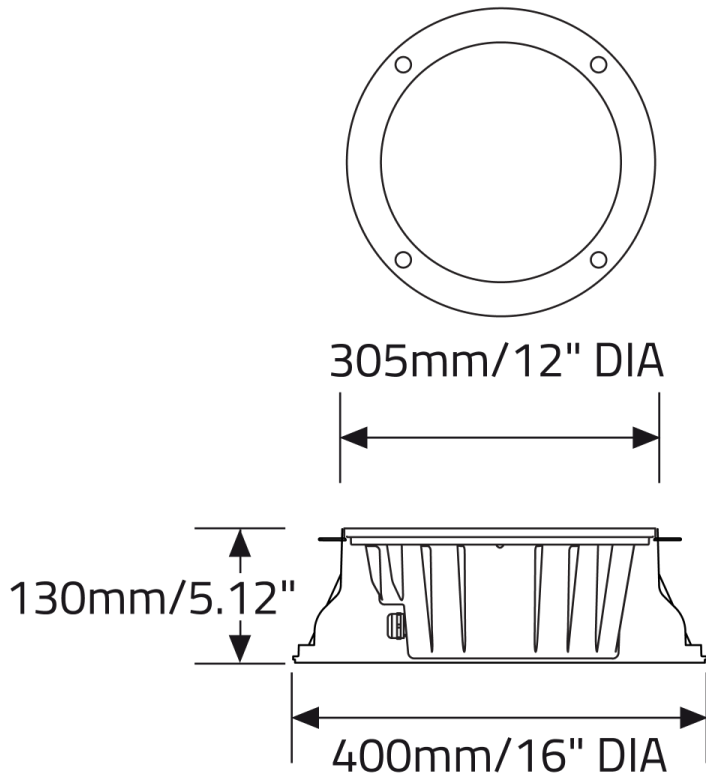
Type A Glass Bezel
